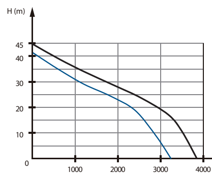
Vesiautomaatti PA-1 Vesiautomaatti PA-2
