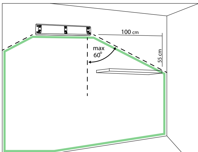
Fig. 1, rätt placering av kroklist
