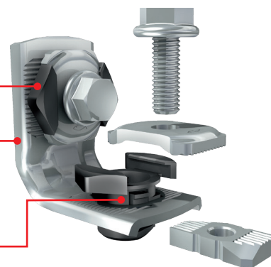
MW Clix 90°
