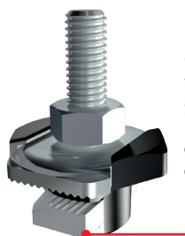
FHS Clix
