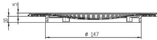
SECTION A-A SCALE 1 : 2
